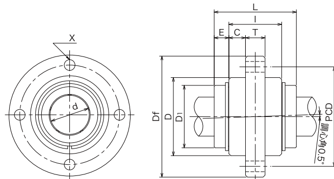
*** 注文番号 PN CD - 12 V UU 呼び番号 | サイズ | 樹脂製リテーナ | 両面シール付 | 中央丸フランジ型
